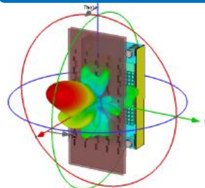
透過型メタサーフェス
