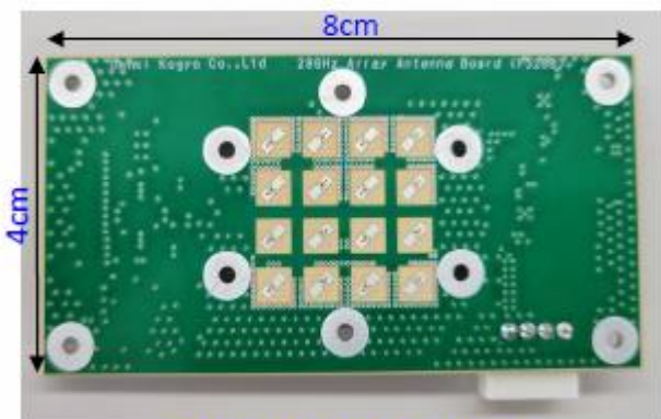
アンテナ(16素子アレー) (表面)
