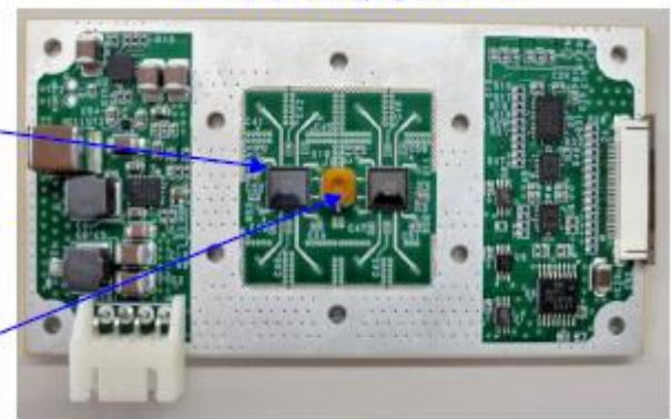
28GHz帯AiP(16素子)(裏面)
